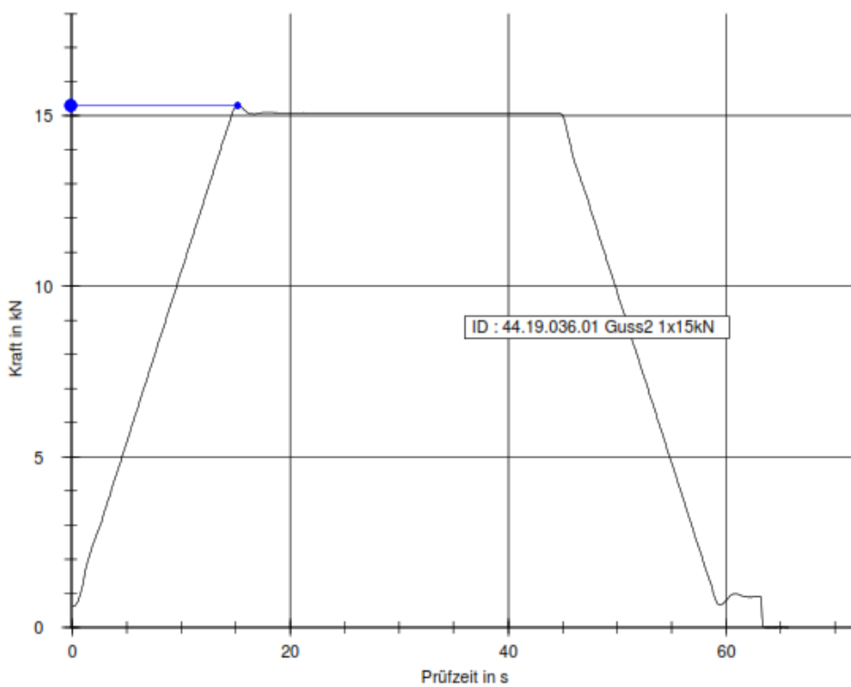
Spécimen 2 : charge de 15 kN durant 30 sec.
